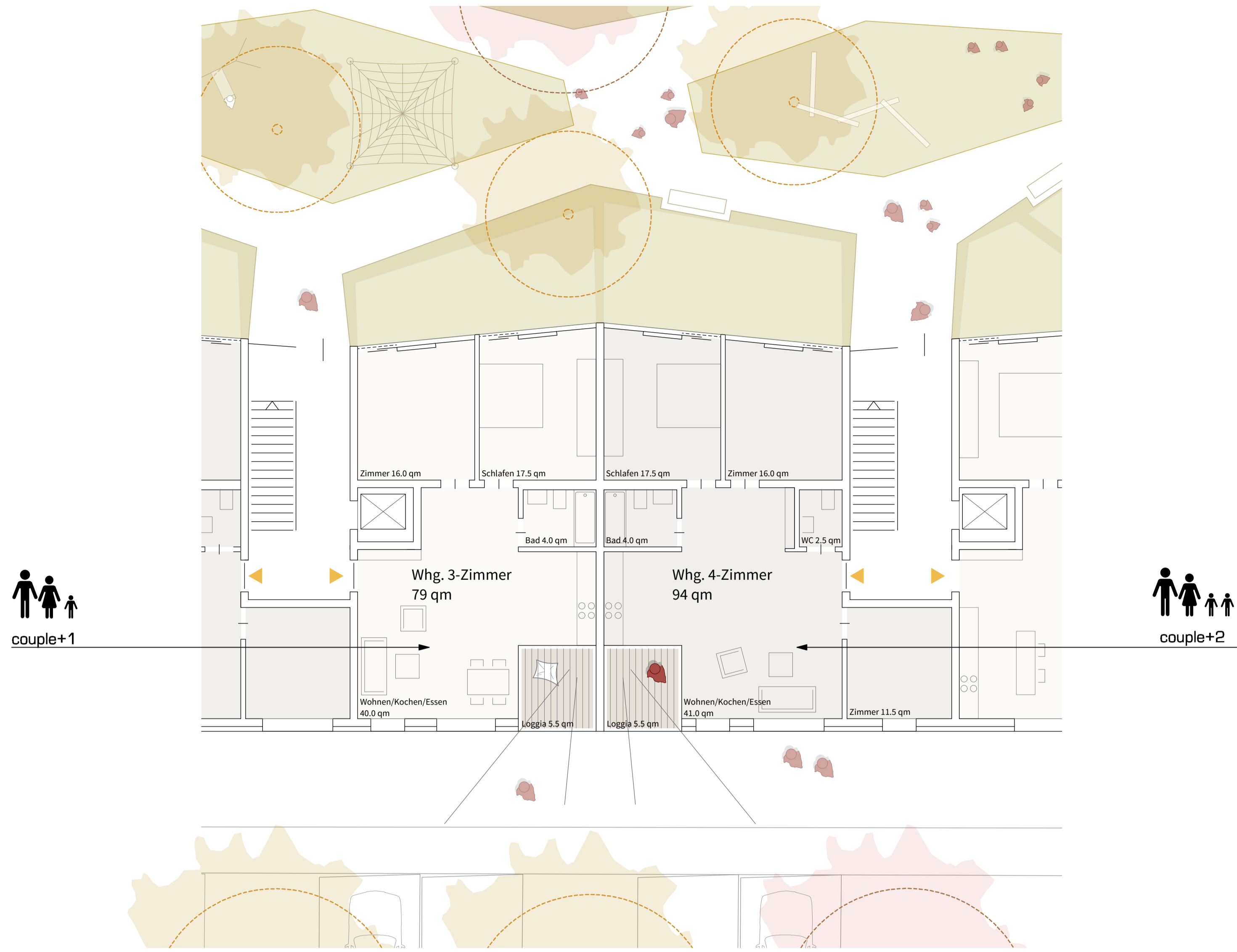
Grundrissausschnitt Wohnung M 1:100
