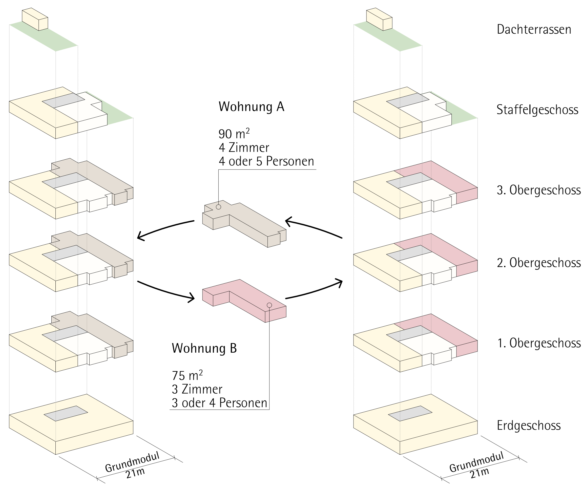
Isometrie - austauschbare Wohnungen
