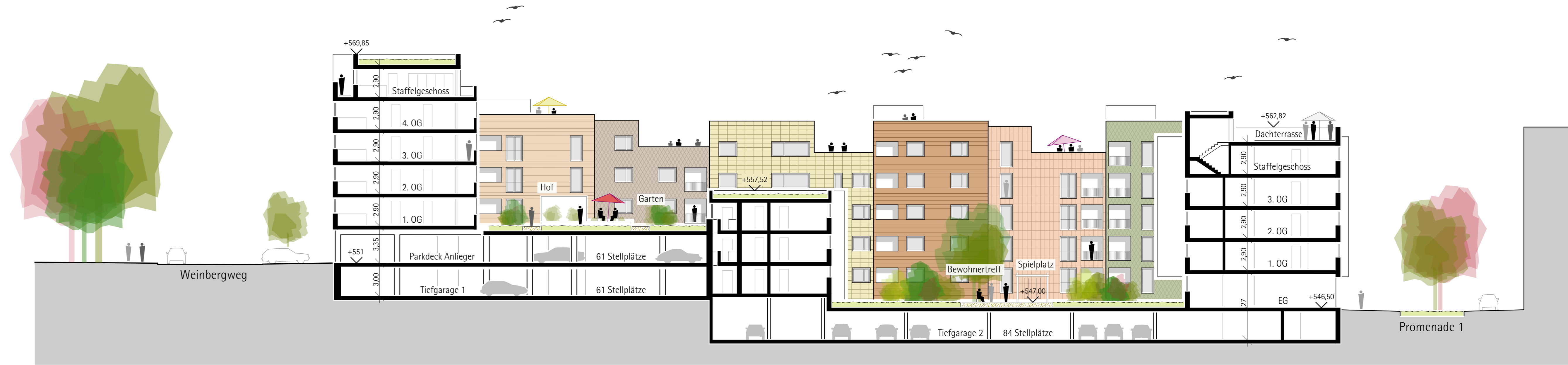
Längsschnitt A-A
