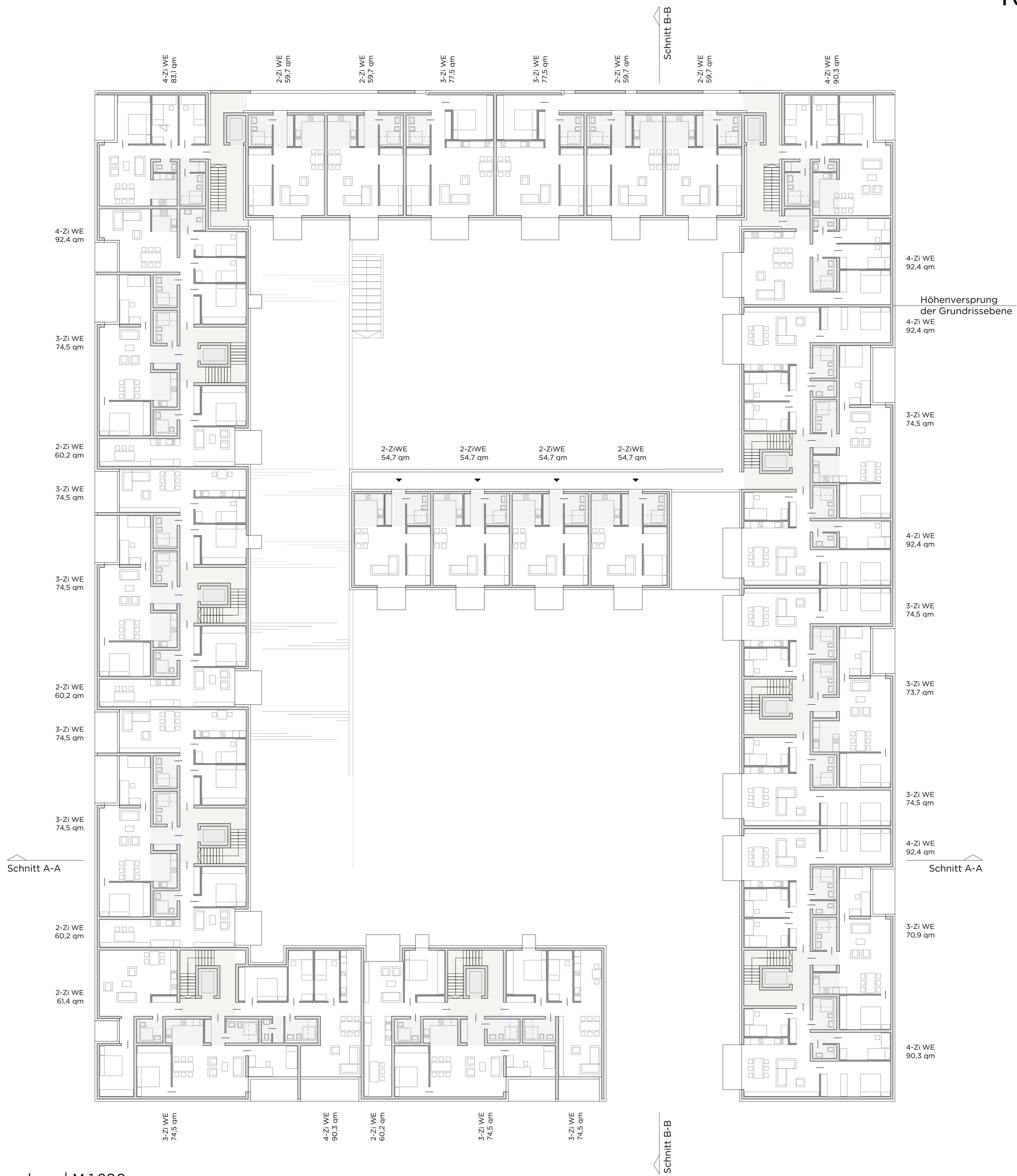
Grundriss 2. Obergeschoss | M 1:200
