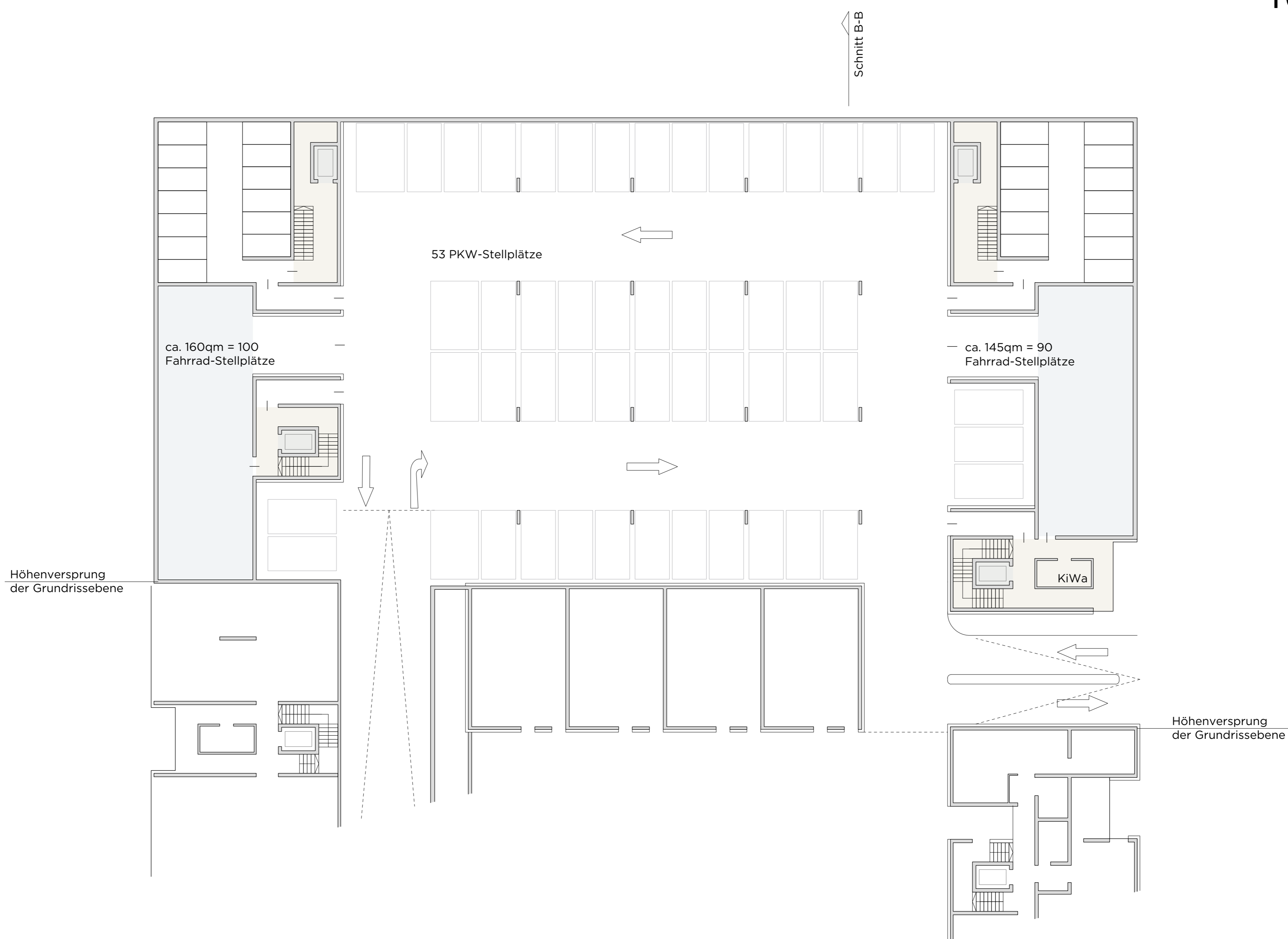
Grundriss Zwischengeschoss UG -1 | M 1:200
