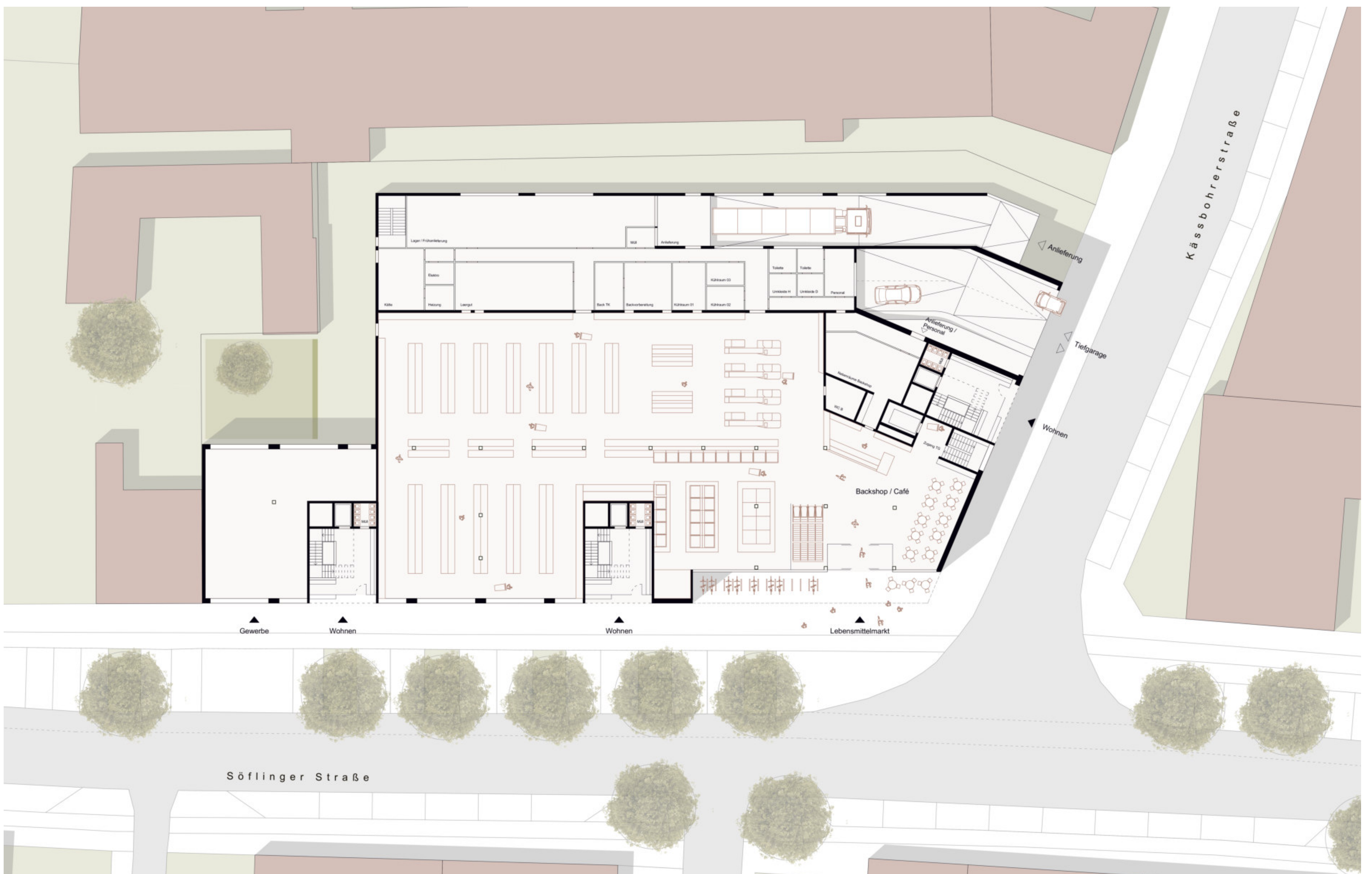
Erdgeschoss 1:200
