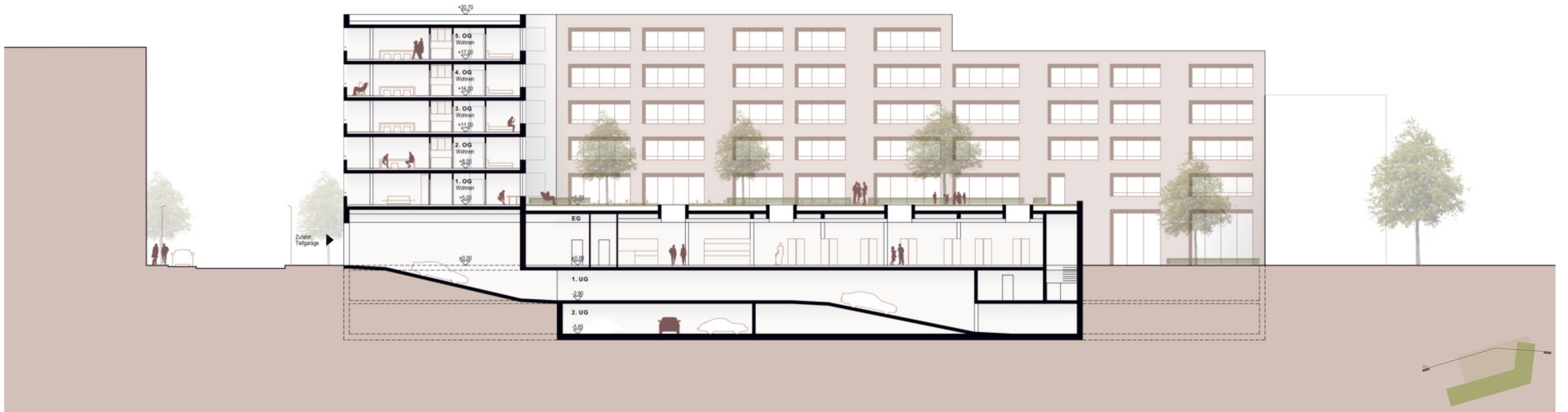
S1 Längsschnitt 1:200
