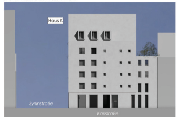
Ansicht Nord, M 1:200
