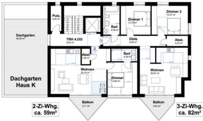
Grundriss 4.OG, M 1:100
