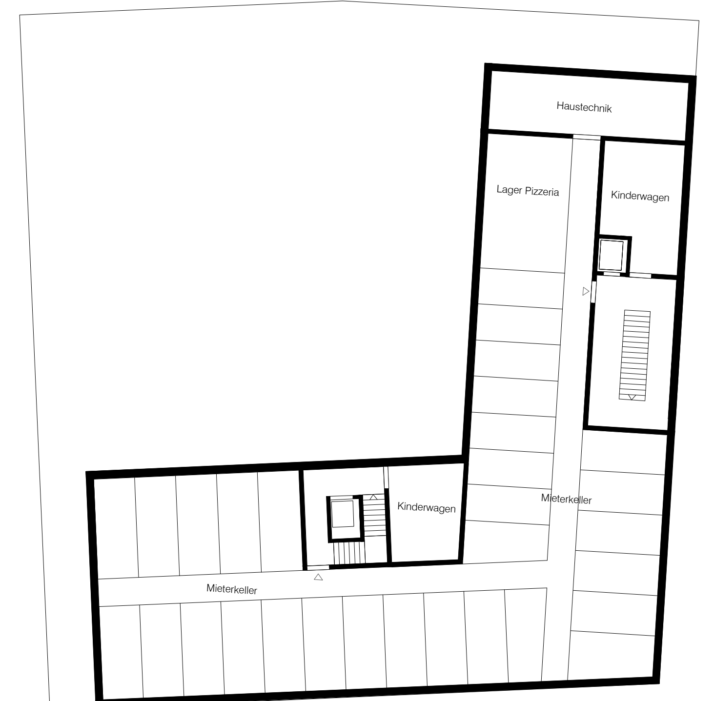
2. Untergeschoss M 1:200
